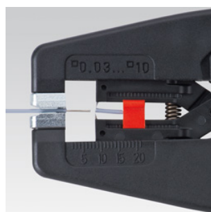
Dénudage précis de 0,03 à 10,0 mm 2 sans réglage
