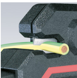
Coupe-fils pour fils jusqu'à 2,5 mm 2 max.
