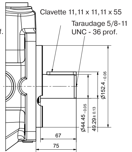
Option de montage F Arbre SAE à clavette
