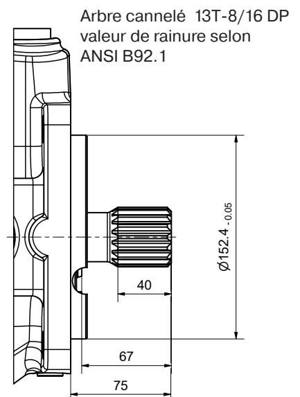
Option de montage G Arbre SAE à clavette
