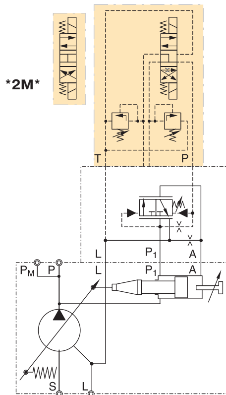
Schéma PVAC2M*/PVAC2E*
