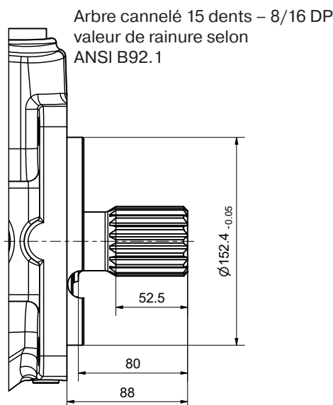
Option de montage E Arbre SAE à clavette
