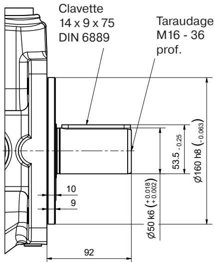
Option de montage Kshaft Arbre métrique à clavette
