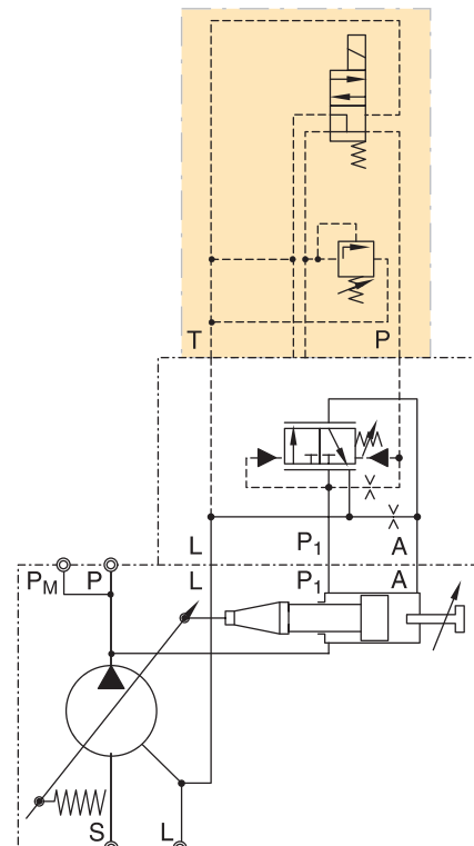
Schéma PVAC1E*
