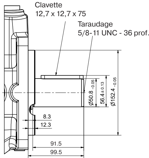
Option de montage D Arbre SAE à clavette
