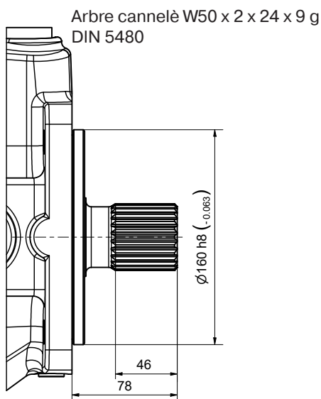
Option de montage L Arbre métrique cannelé
