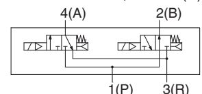
Distributeur 2x4/2, 3 voies (C)
