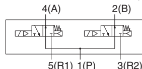
Distributeur 3x3/2, 4 orifices (B)
