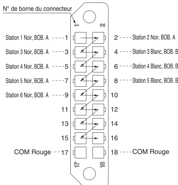
Exemple de spécifications d'embase
