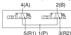
Distributeur 2x4/2, 3 orifices (A)
