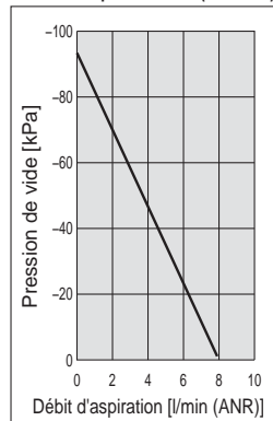
Caractéristiques du débit (0.45 MPa)
