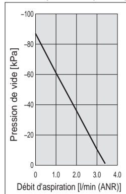
Caractéristiques du débit (0.35 MPa)
