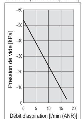
Caractéristiques du débit (0.45 MPa)
