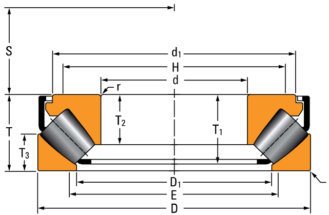
Type TSR-EJ
