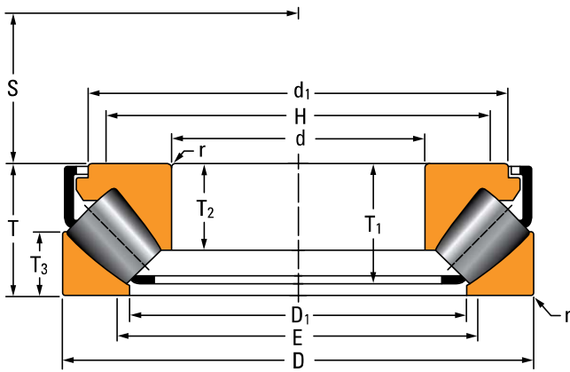
Type TSR-EJ
