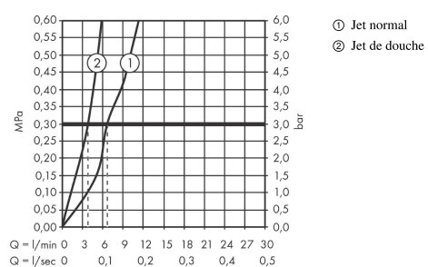
Schéma d'écoulement
