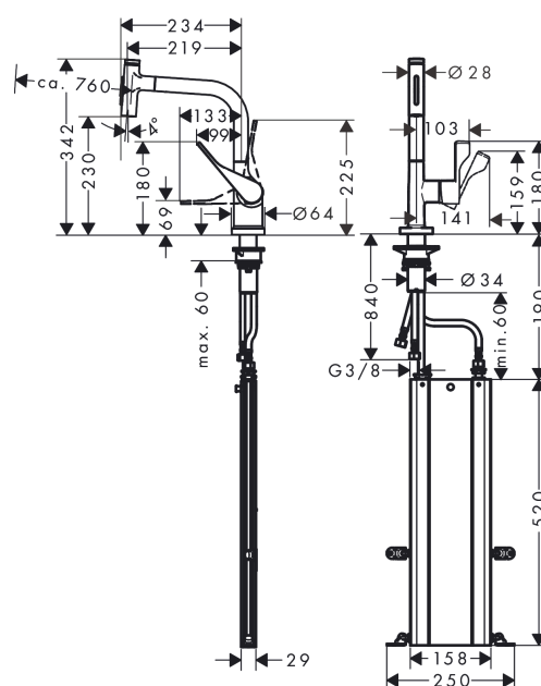
Plan géométral
