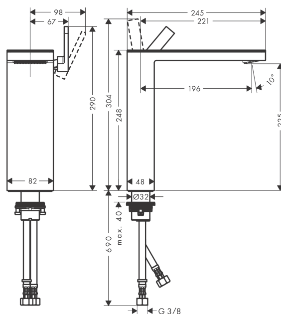
Plan géométral
