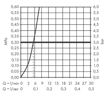
Schéma d'écoulement
