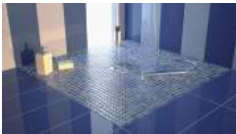
Un panneau hydrofuge prêt à carreler avec pente intégrée
