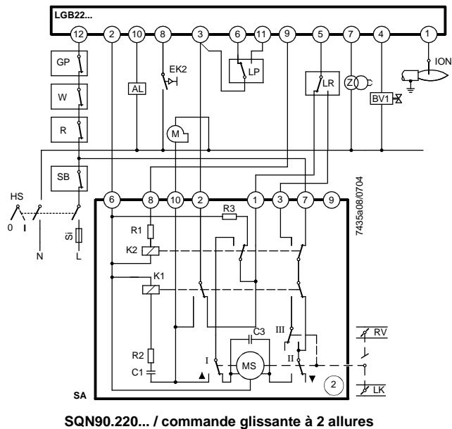
SQN90.220... / commande glissante à 2 allures
