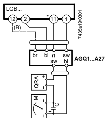
Circuit de mesure
