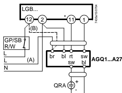
Schéma de raccordement
