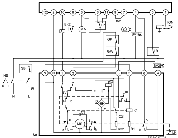
SQN91.140... / commande à 2 allures
