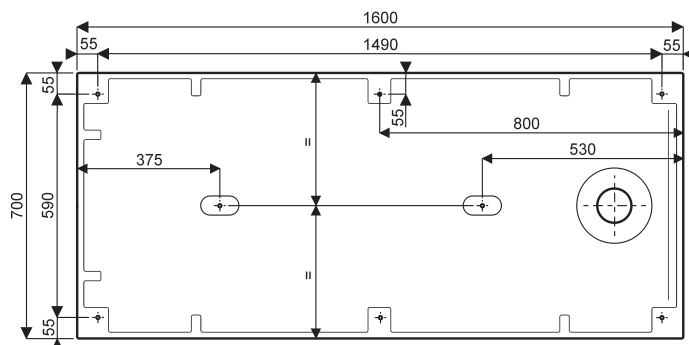
000946 00 xxx Receveur extra-plat rectangulaire 160 x 70 en MARBEX® à poser ou à encastrer, pour bonde siphon de 90.
