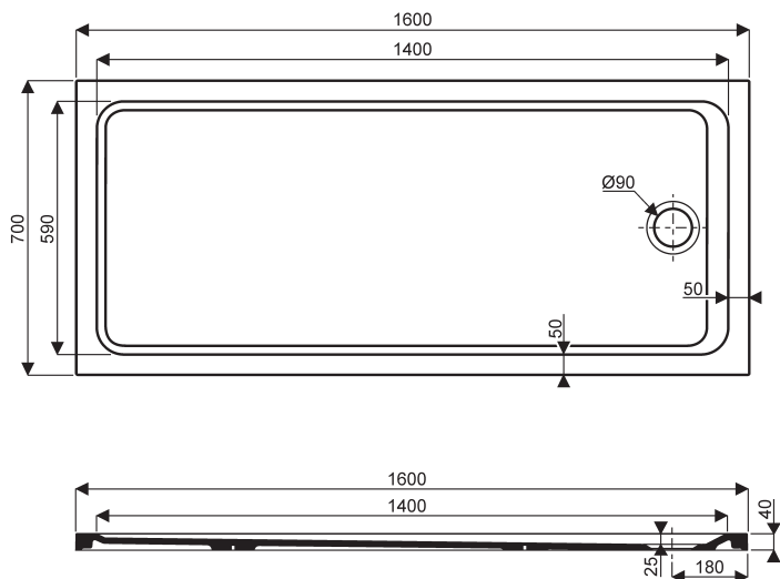
000946 00 xxx Receveur extra-plat rectangulaire 160 x 70 en MARBEX® à poser ou à encastrer, pour bonde siphon de 90.
