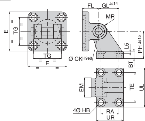
MP2 + AB7 Chape arrière démontable + Tenon arrière démontable
