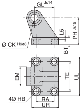
FIXATION ARRIÈRE Tenon arrière démontable AB7
