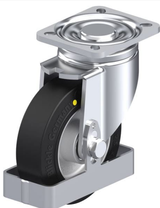
Roulette pivotante correspondante LH-ALEV 125K-1-EL-FS
