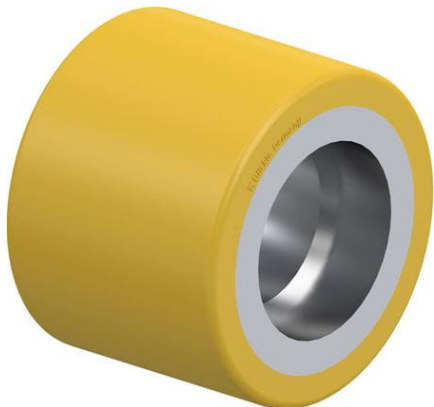
Roulette associée (sans roulement à billes) RK-HTH 080x062/47x18-62-Z
