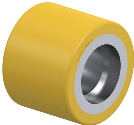
Roulette associée (sans roulement à billes) RK-HTH 082x070/47x14-70-Z
