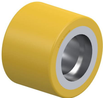
Roulette associée (sans roulement à billes) RK-HTH 082x070/47x12-70-Z
