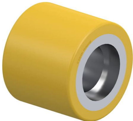
Roulette associée (sans roulement à billes) RK-HTH 082x072/47x14-72-Z
