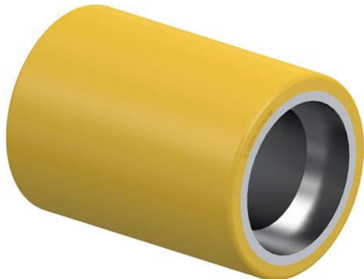
Roulette associée (sans roulement à billes) RK-HTH 083x083/52x15-83-Z
