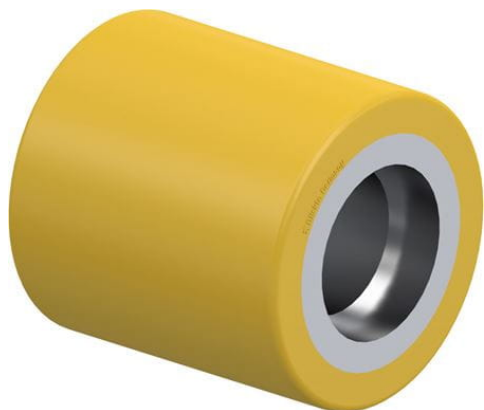
Roulette associée (sans roulement à billes) RK-HTH 085x110/47x14-110-Z
