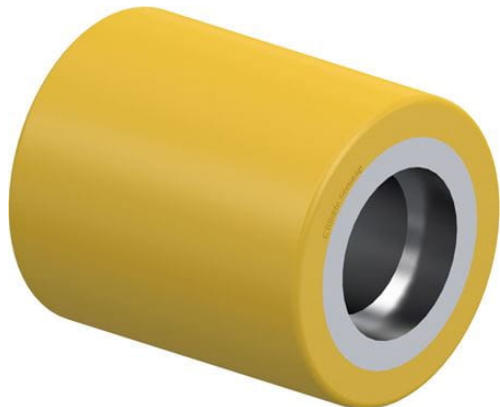
Roulette associée (sans roulement à billes) RK-HTH 085x050/47x14-50-Z
