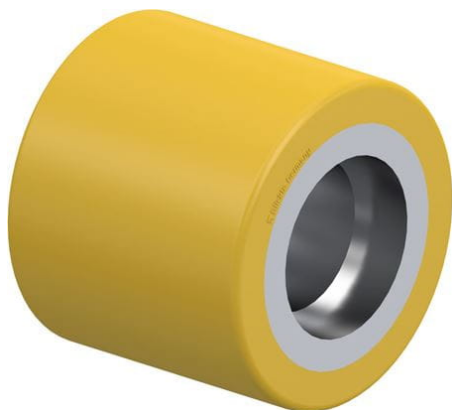
Roulette associée (sans roulement à billes) RK-HTH 085x085/47x14-85-Z
