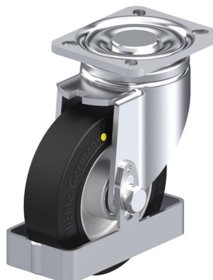
Roulette pivotante correspondante LH-ALEV 125K-1-EL-FS
