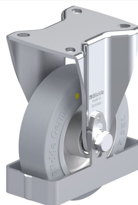
Roulette fixe correspondante BH-ALEV 125K-1-SG-AS-FS
