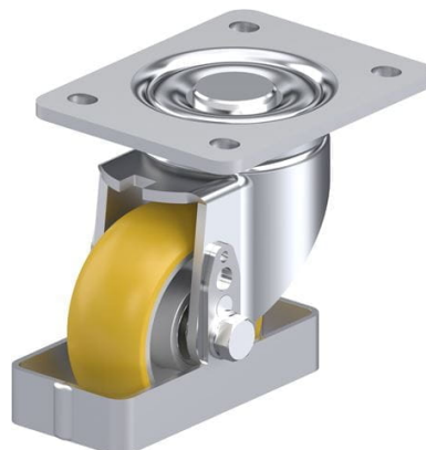
Roulette pivotante correspondante LH-ALTH 101K-3-CO-FS
