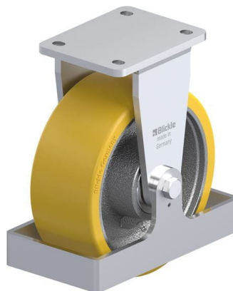
Roulette fixe correspondante BO-GTH 202K-FS
