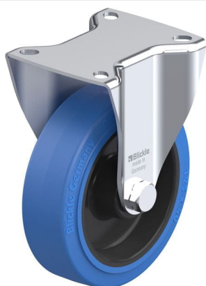
Roulette fixe correspondante BK-POEV 125XR-1-SB
