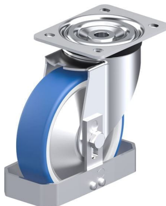
Roulette pivotante correspondante L-POTHS 160K-FA-FS
