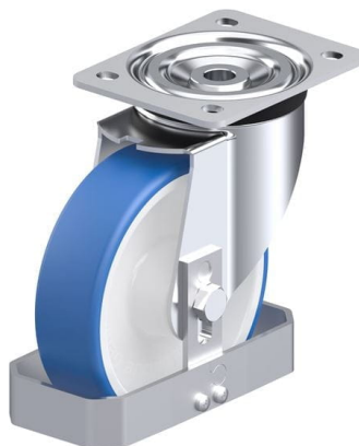
Roulette pivotante correspondante L-POTHS 160R-FS
