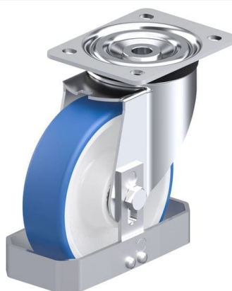
Roulette pivotante correspondante L-POTHS 160XK-FS
