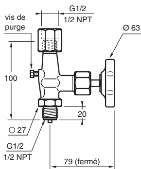
Robinet à pointeau
