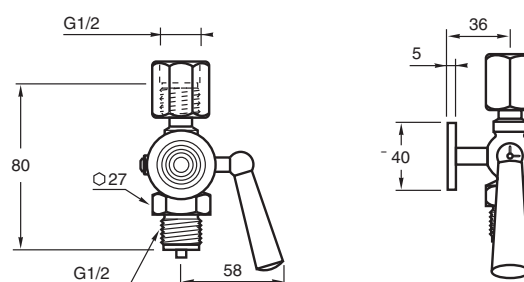
Robinet à boisseau avec bride de contrôle
