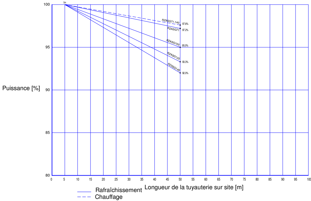
Puissance en fonction de la longueur de tuyauterie sur site
