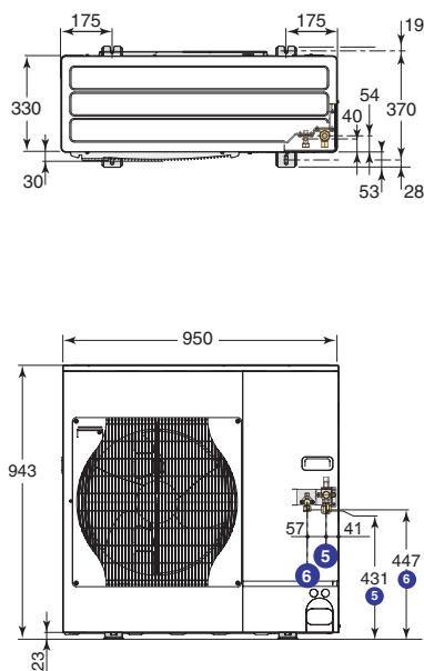
AWHP 8 MR-2
