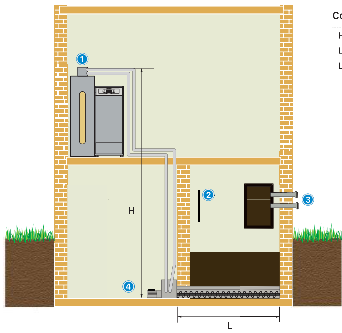
Vis sans fin motorisée pour alimentation silo artisanal 1,5 TKITBIO058
