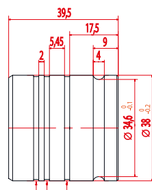
Gorges pour circlips ext. Ø 38 DIN 471 & AFNOR NF E 22-163 Grooves for 38 mm dia. external circlips to DIN 471 & AFNOR NF E 22-163
