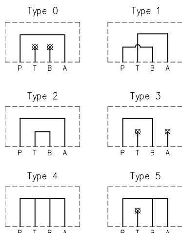
Schémas hydrauliques
