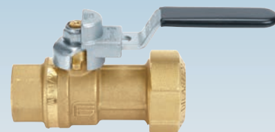
art. 4E03...P F/TOF levier en acier avec possibilité d'application de cadenas, plastifié noir (Blocage ON et OFF) H/TOF palanca de bloqueo de acero plastificada negra (bloqueo ON y OFF)
