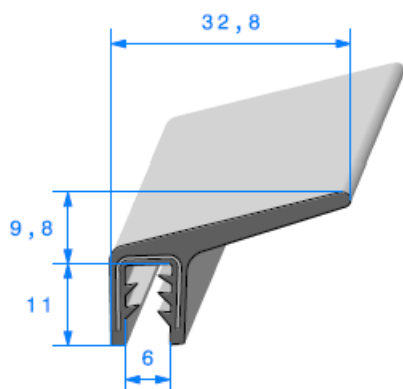
Dessin du profil
