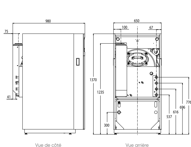
Axeo NOx F07 / Axeo NOx F30
