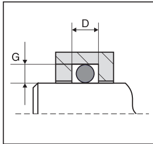
Figure 5 montage piston / alésage
