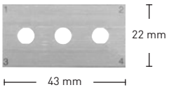
REF 135.2 Ep. 0,2 mm Lame en acier supérieur.
