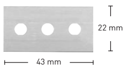
REF 435.3 ALD Ep. 0,3 mm Lame en acier inox alimentaire.
