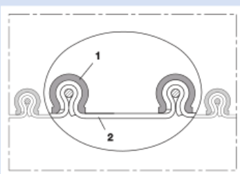
Tuyau PVC avec profilé de serrage (tuyau clippé) (jusqu'à +120°C)
