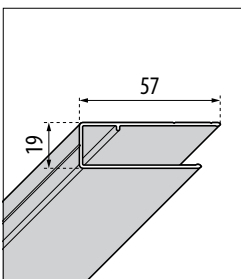
VERBREDINGSPROFIEL PROFILÉ D'ÉLARGISSEMENT
