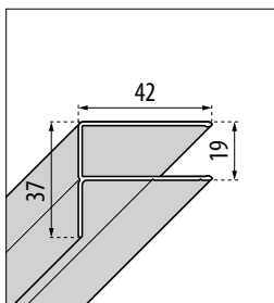
MUURPROFIEL PROFILÉ MURAL
