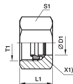
X1) Bague d'ancrage
