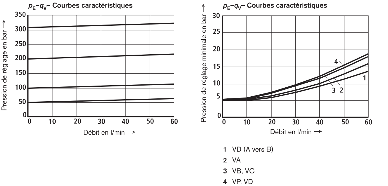
Courbes caractéristiques correspondant à la pression atmosphérique à la sortie sur toute la plage de débit!
