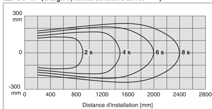
IZF31-W (Avec louvre réglable : Paramètre d'angle 5, Niveau du débit d'air : 10)
