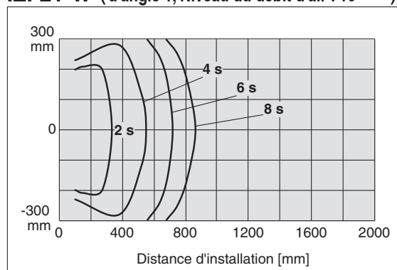
IZF21-W (Avec louvre réglable : Paramètre d'angle 1, Niveau du débit d'air : 10)
