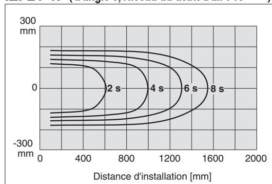
IZF21-W (Avec louvre réglable : Paramètre d'angle 5, Niveau du débit d'air : 10)
