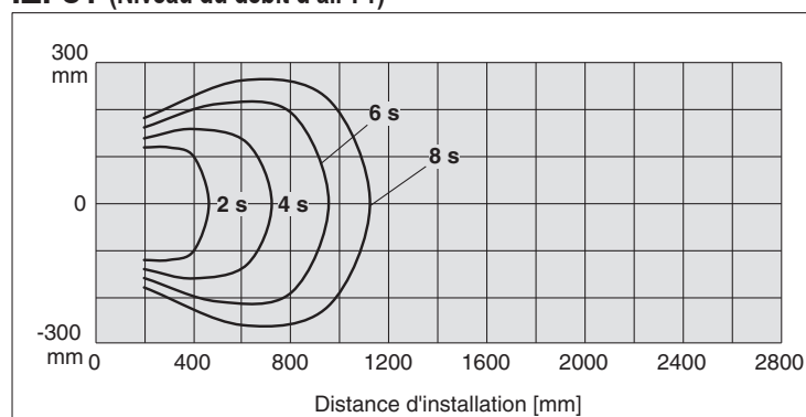
IZF31-W (Avec louvre réglable : Paramètre d'angle 1, Niveau du débit d'air : 10)
