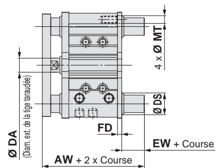
Vérin avec racleurs des deux côtés
