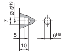
Schéma détaillé de coupe XX
