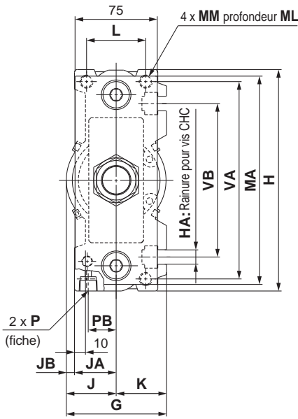
Schéma détaillé de coupe XX
