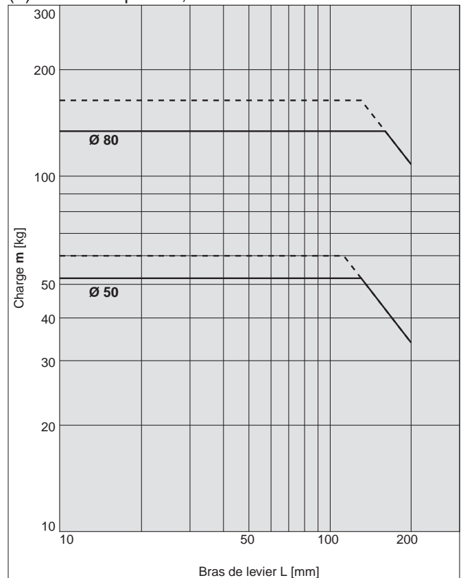
(4) Course sup. à 50, V = 400 mm/s
