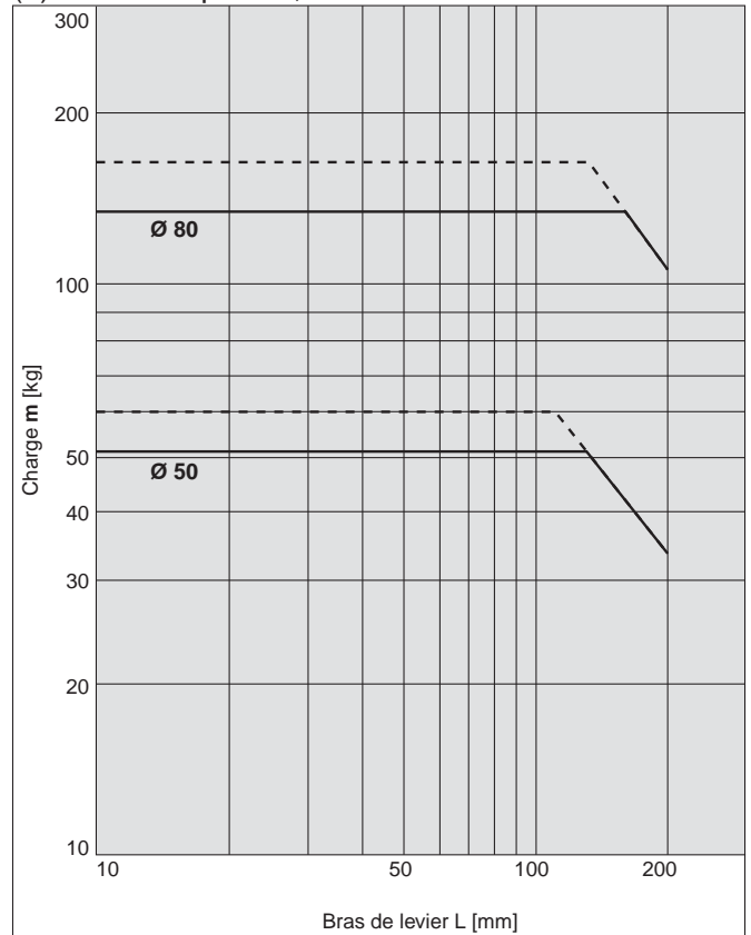
(2) Course sup. à 50, V = 200 mm/s max.
