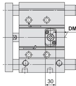
Avec verrouillage arrière
