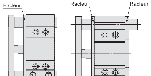
Racleur d'un seul côté
