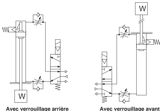
Avec verrouillage arrière
