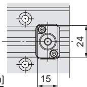
Ø 25 Mécanisme de verrouillage de tige (Déverrouillage bistable)
