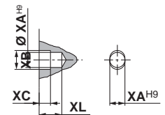
Schéma détaillé de coupe XX
