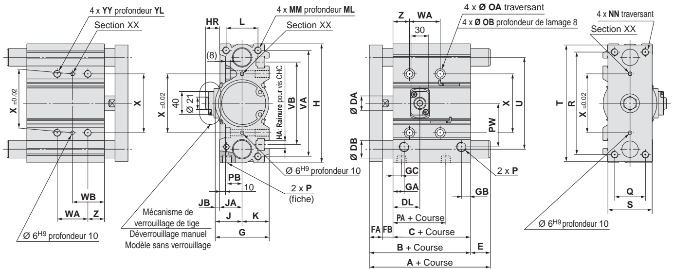
Avec verrouillage avant
