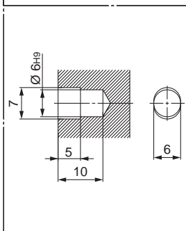
Détails de la section XX
