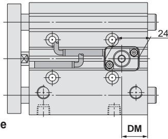
Avec verrouillage arrière
