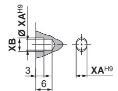
Schéma détaillé de coupe XX
