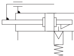
Symbole Amortissement élastique
