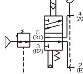
Régulation de l'orifice A
