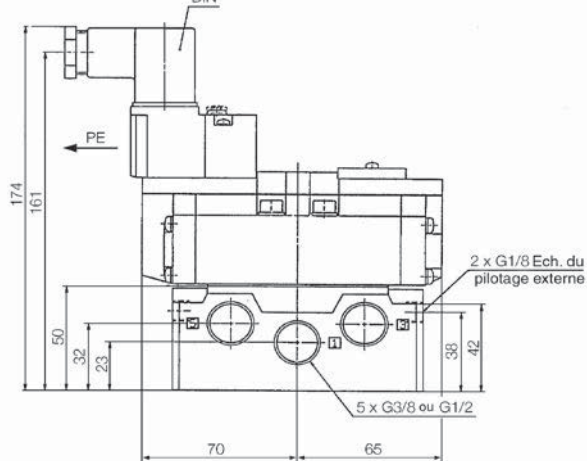
EVS7-8-FG-S-□CV-Q
