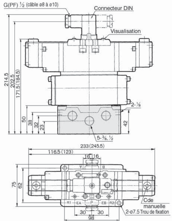
VS7-8-FPG-□□ Orifice de l'embase -Q
