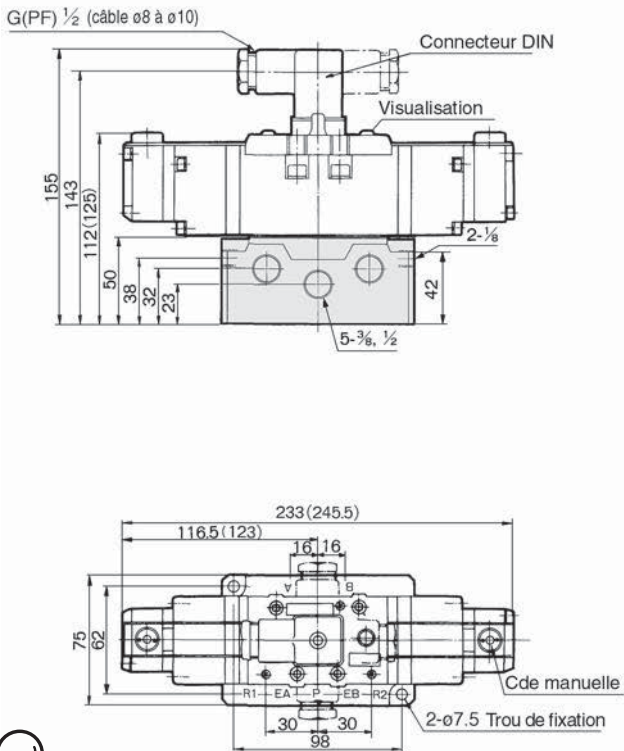
VS7-8-FJG-□□ Orifice de l'embase -Q
