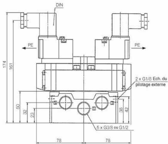
EVS7-8-FHG-D-□CV-Q • EVS7-8-FJG-D-□CV-Q • EVS7-8-FIG-D-□CV-Q
