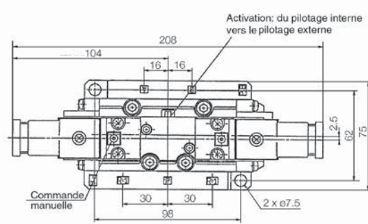
EVS7-8-FHG-D-□CV-Q • EVS7-8-FJG-D-□CV-Q • EVS7-8-FIG-D-□CV-Q
