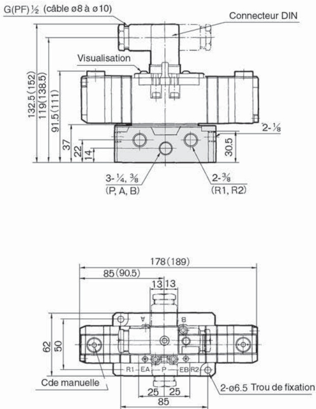
VS7-6-FJG-□□ Orifice de l'embase -Q
