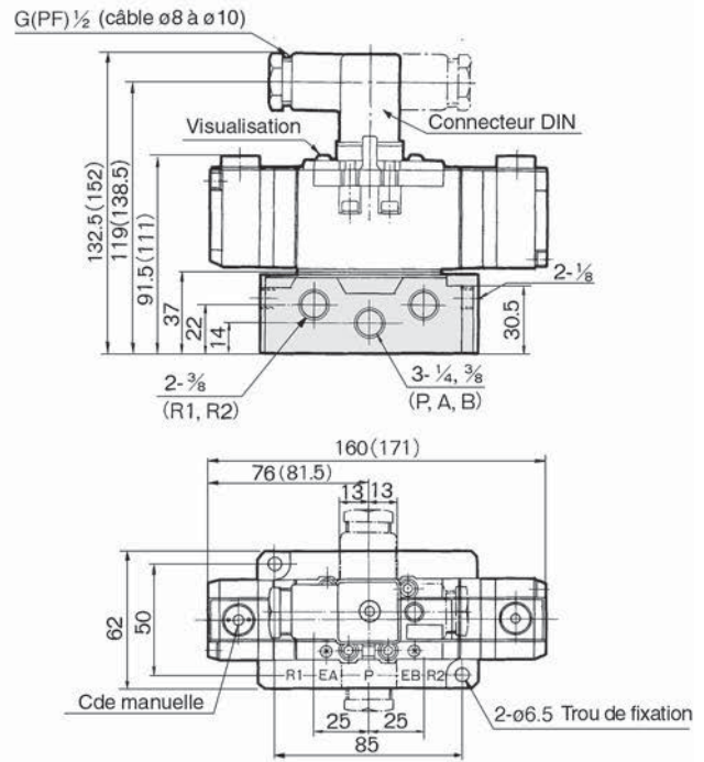
VS7-6-FPG-□□ Orifice de l'embase -Q
