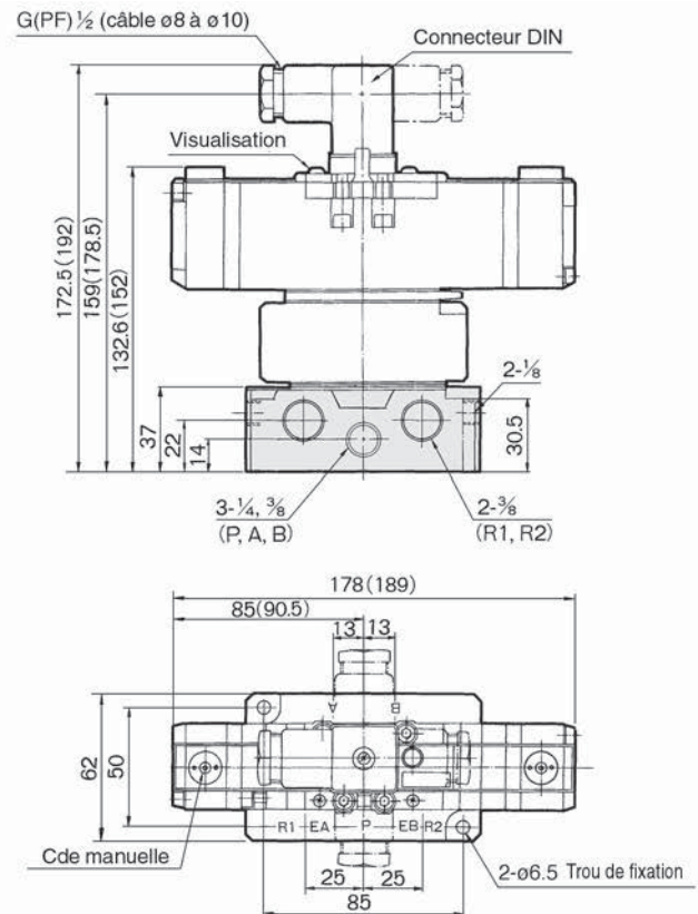
VS7-6-FPG-□□ Orifice de l'embase -Q
