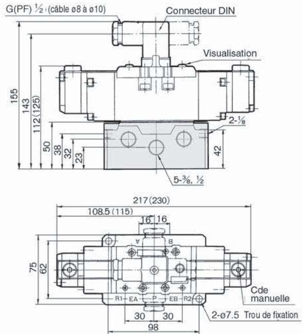
VS7-8-FPG-□□ Orifice de l'embase -Q
