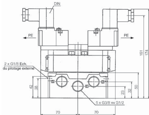
EVS7-8-FG-D-□CV-Q
