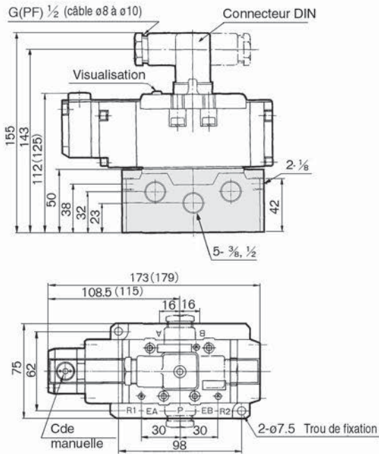
VS7-8-FHG-□□ Orifice de l'embase -Q
