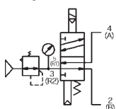
Régulation de l'orifice P
