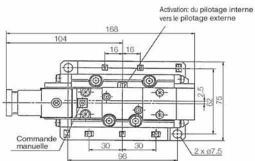
EVS7-8-FHG-D-□CV-Q • EVS7-8-FJG-D-□CV-Q • EVS7-8-FIG-D-□CV-Q
