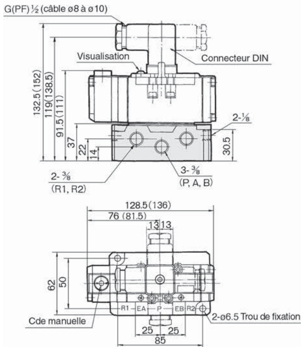
VS7-6-FHG-□□ Orifice de l'embase -Q
