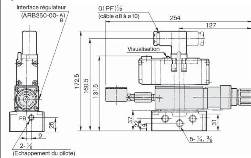
Régulation de l'orifice A/ARB250-00-A Régulation de l'orifice B/ARB250-00-B
