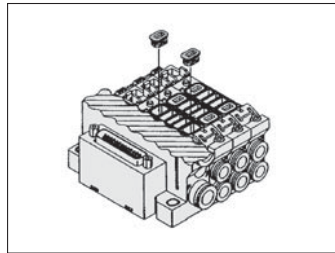
Clapet anti-retour de contre-pression [-B] VVQ2000-18A
