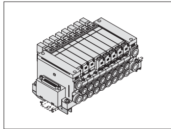
Fixation de montage pour rail DIN [-D/-D0/-D□] VVQ2000-57A
