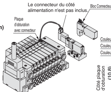
Passage ALIM. bloqué
