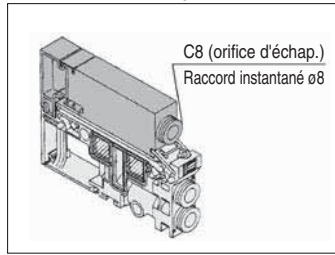
Entretoise d'échap. individuelle VVQ2000-R-1-C8 N9
