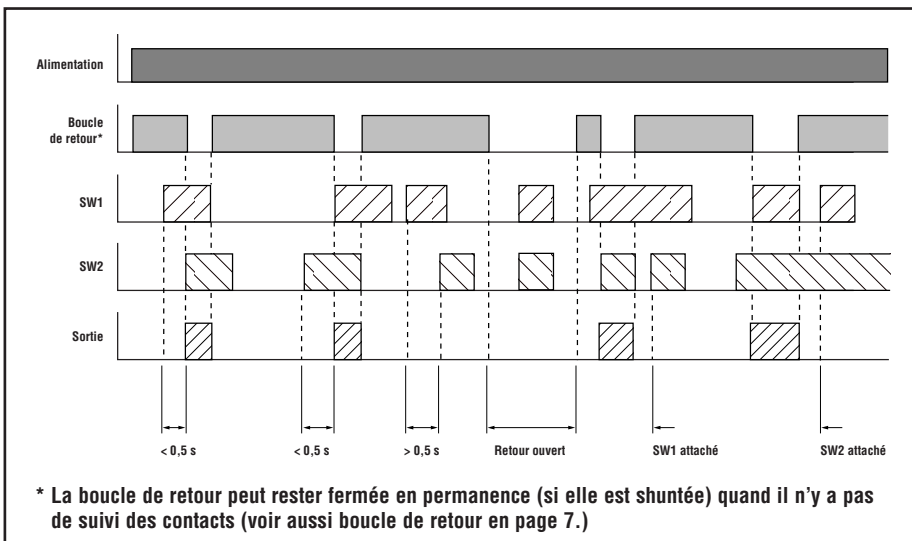
Figure 2. Diagramme de temps du module de sécurité DUO-TOUCH SG AT-FM-10K
